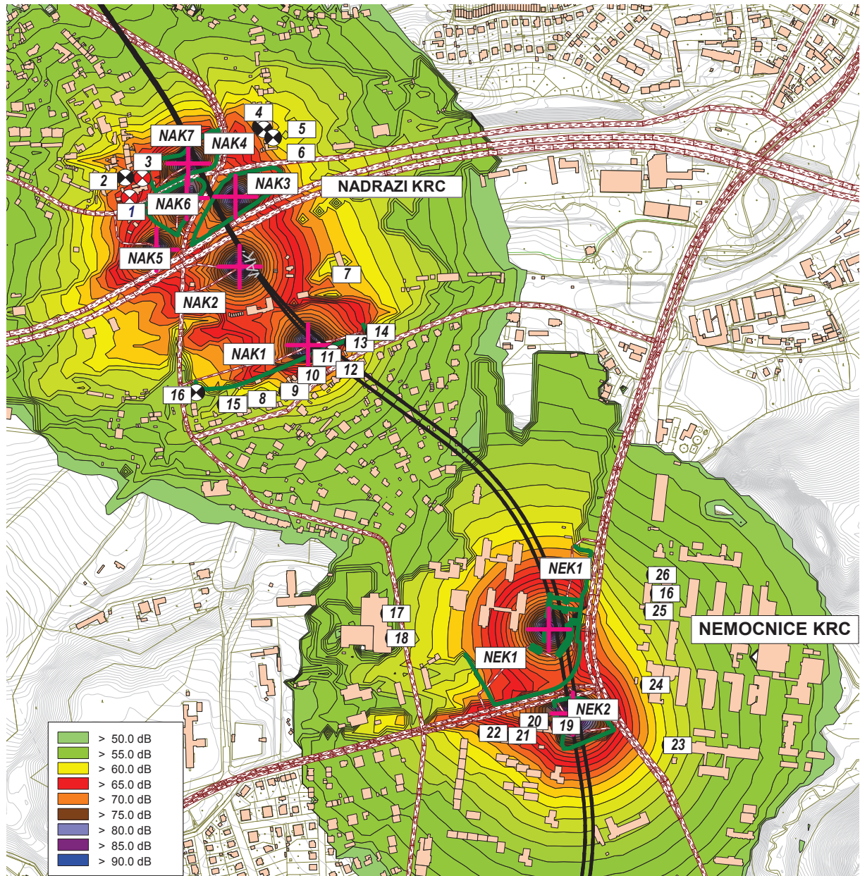
Obr. č. 37 Průběh izofon – hluk ze stavební činnosti v okolí stavenišť NAK 1-7 a NEK 1,2
