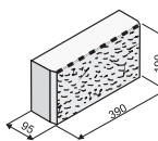
Tvarovka štípaná přizdívací
