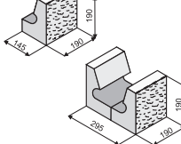
Tvarovka věncová štípaná - půlená pro řadu šíře 300
