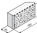
Tvarovka štípaná zkosená
