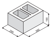
Tvarovka hladká dělitelná
