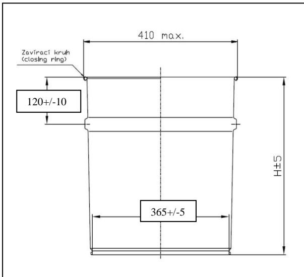
Rozměry sudu
