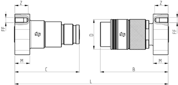
Flange Adapter - Adattatore con Flangia - Flanschadapter - Reccordement Bride (ISO 6162-2)
