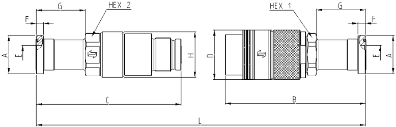
Flange Head Adapter - Codolo per Flangia - Flanschtelleradapter - Fixation raccordement Bride (ISO 6162-2)
