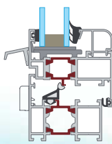
Okno otvíravé – fez
